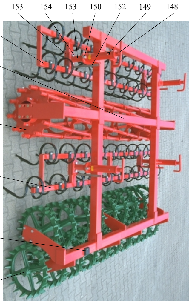
Abb. 14 Seitenrahmen in Fahrtrichtung rechts
